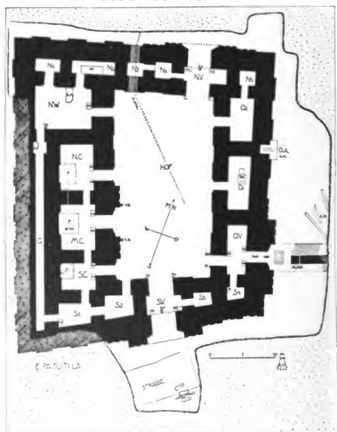
FIG. 142.—Plan of Epatutilla.
