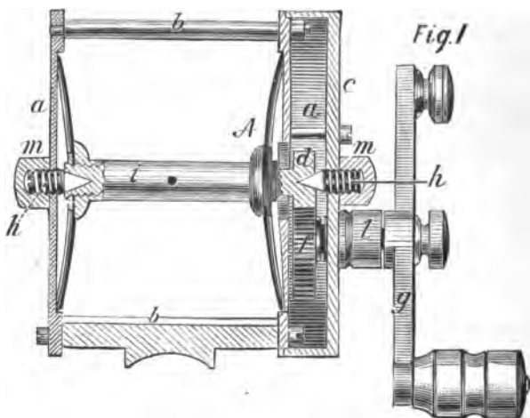
"Imbrie" Compensating Reel. (Abbey & Imbrie.)
