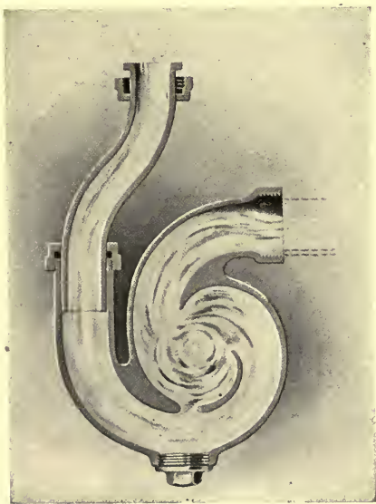
FIG. 45.—Non-siphoning trap vent, "Sanito" model (J. L. Mott Co.).
