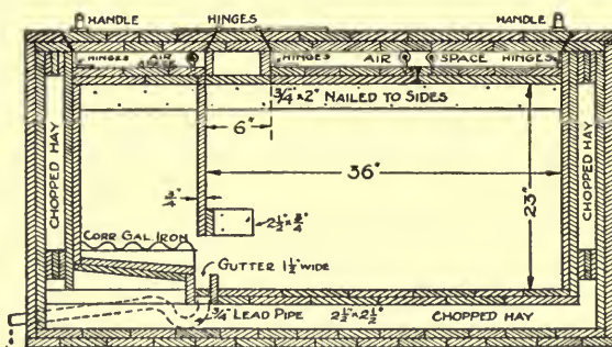
LONGITUDINAL SECTION
