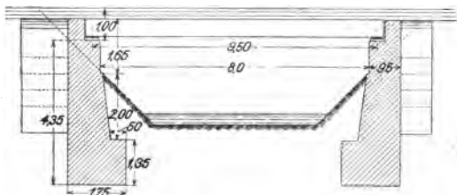
Schnitt a-b.
