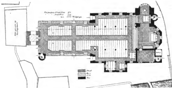
Grundriß zur Erweiterung der Stadtpfarrkirche in Haslach i. K.
