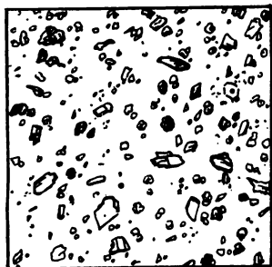
FIG. 28.—Terra Alba.
