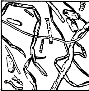
FIG. 44.—Straw.
