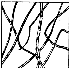
FIG. 36.—Linen.
