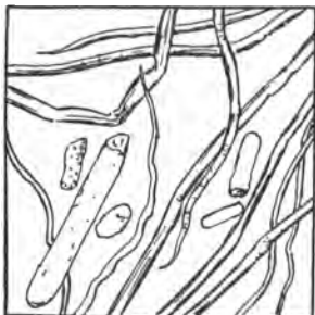
FIG. 47.—Bamboo.
