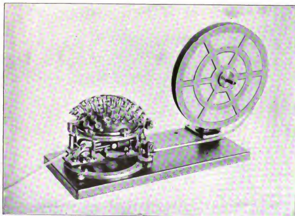
Schreibmaschine von Welling-Hansen 1872
