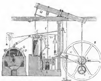
Eine alte Dampfmaschine zur Zeit des Todes von James Watt
