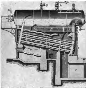
3. Wasserrohrkessel mit Überhitzer; E Feuerzug, W Wasserrohre, K Wasserkammern, Z Zylinder- kessel, S Dampfsammler, U Überhitzer, L Dampfleitung, Sp Speiseventil, Si Sicherheitsventil, w Wasserstandsglas mit Manometer m, C Schornsteinkanal.
