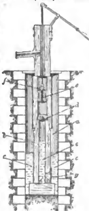
Saugbrunnen.
