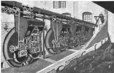
6. Automatische Feuerung. Weg der Kohle K: durch die Rinne R mittels Transportschraube zum Elevator E, von da in der Verteilerrinne V mittels Transportschraube S zu den Trichtern I; weiterer Weg: Fig. 7.
