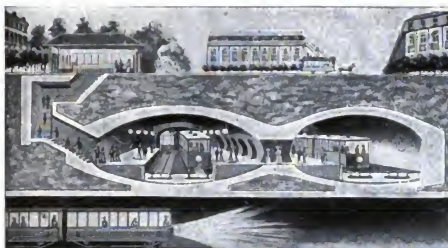
2. Pariser Untergrundbahn (Querschnitt an der Place de l'Étoile).
