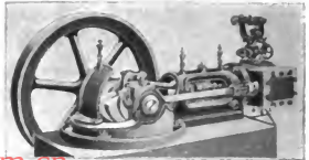
2. Einzylindermaschine mit Schlebersteuerung.
