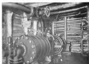
5. Mehrstufige Zentrifugalpumpe für Grubenbetrieb (elektrischer Antrieb).
