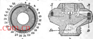
Brennzünder: a Sackhül von unten, b Längsschnitt.
