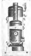
2. Querrohrkessel; F Feuerzug, Q Quer- rohre, S Schornstein, L Dampfleitung, W Wasserstandglas, G Reinigungs- öffnungen.
