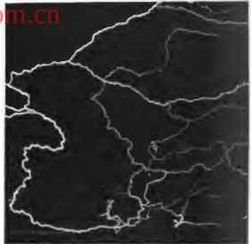
6. Linienblitz, nach einer Photographie von P. Liebig.
