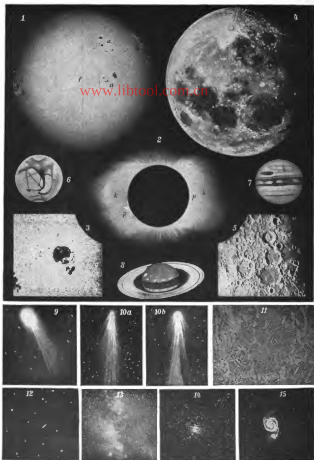
1. Sonne (nach Photogr. von Lohse in Potsdam); a Flecken; b Fackeln; f Orientierungsfaden im Fernrohr. 2. Sonne während der totalen Verfinsternung nach Photogr. der Expedition der Smithsonian Institution zu Wadesboro Nordkarolina, 28. Mai 1900; k , p Protuberanzen. 3. Sonnenfleck und Granulation eines Teiles der Sonnenoberfläche (nach Photogr. in Meudon, 2. Juni 1856). 4. Mond (nach Photogr. von Hartmann in Potsdam, 10. Juni 1880). 5. Teil der Mondoberfläche (nach Photogr. von Loewy und Paiseux in Paris). 6. Merkur (nach Zeichn. von Schiaparelli). 7. Jupiter mit dem roten Fleck (nach Zeichn. von Lohse). 8. Saturn (nach Zeichn. von Trouvelot in Cambridge, Mass.). 9. Komet 1907 d (Daniel (nach Photographie). 10. Komet 1908 c Morehouse, a aufgenommen am 10. Nov., b am 16. Nov. 1908. 11. Widmanstätten'sche Figuren, auf Meteoriten erzeugt. (8. Meteorstein). 12. Planetoid, der sich als Lichtstrich von den Fixsternen (Lichtpunkten) abhebt. (8. Planeten). 13. Milchstraße, Mitte 9 Vulpeculae (nach Aufnahme von Wolf in Heidelberg). 14. Sternhaufen im Antinous (nach Photogr. von Roberts). 15. Spiralebel in den Jagdhunden (nach Photogr. von Ritchey, Yerkes-Sternwarte).
