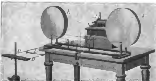
10. Erzeugung stehender Elektrischer Wellen (s. d.); F Funkeninduktor, K Funkstrecke, D Drahte, B Drahtbügel, L Lechersche Röhre.
