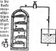
Ammoniak: Apparat zur Darstellung von Ammoniak aus Stickstoff nach Frank (schematisch).
