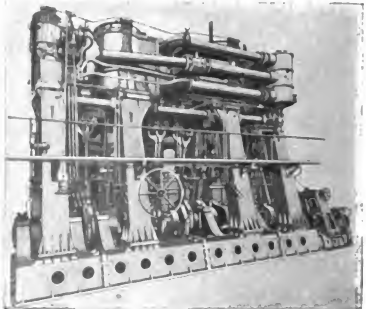
9. Vierzylindrige Vierfach-Expansions-Schiffsmaschine.
