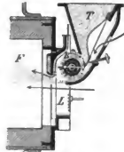
4. Staubfeuerung; F Einfeldtrichter für die Staubkohle, B rotierende Bürste, F Feuerraum, L Luftschieber.
