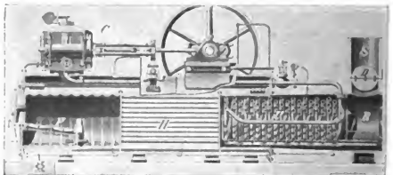
6. Halblokomobile; F Feuerung, H Heizrohren, U Überhitzer, R Rauchkammer, S Schornstein, D Drosselklappe, C Verbundmaschine.
