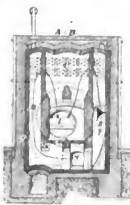
1. Etzflamrohrkessel mit Überhitzer (Querschnitt A-B und Längsschnitt); 1, II, III Flammrohr und 1., 2. und 3. Feuerzug; F Feuerzug; NW Normalwasserstand; D Dampfdom, von dem der Dampf über E und M nach Überhitzer U und von hier über N nach Dampfventil V geht; L Sicherheits-, S Speiseventil; H Ablahnh, C Fuchs.
