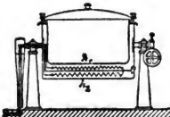
Elektrische Kochapparate: Kippröhrer Kocher der Siemens-Schuckert-Werke für Großküchen (Schematisch).
