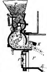
7. Automatische Feuerung: T Einfeldtrichter, S rotierende Speisewalze, W Wurfgewölbe mit Wurfrad r, K schwingende Verteilungsklappe, F Feuer- raum mit Rost R, f Feuertr.
