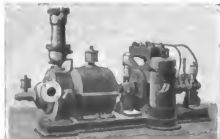
7. De Laval'sche Dampfturbine (7), eine Dynamomaschine (D) treibend.
