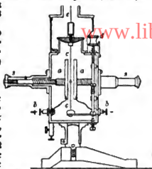
Elektrometer nach Wien (aus H. Schmidt, „Probleme der modernen Chemie“).
