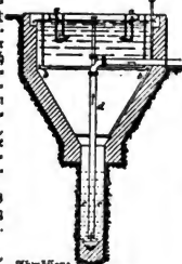
Abwasser: Klärbrunnen nach Kremer.
