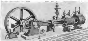
3. Tandemmaschine; H Hochdruck, N Niederdruckzylinder.
