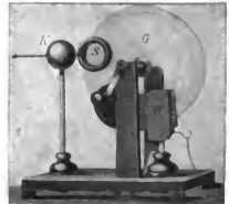
4. Winters Reibungselektriermaschine; G Glasscheibe, R Reibkissen, S Saugapparat, K Konduktor.
