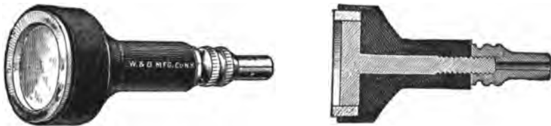
FIG. 126.—UNPOLARIZABLE ELECTRODE.
