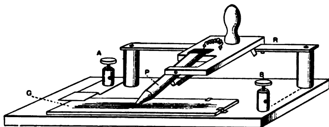
FIG. 106.—GRAPHITE PENCIL RHEOSTAT.
