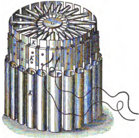
FIG. 73.—THE NOË THERMOPILE.
