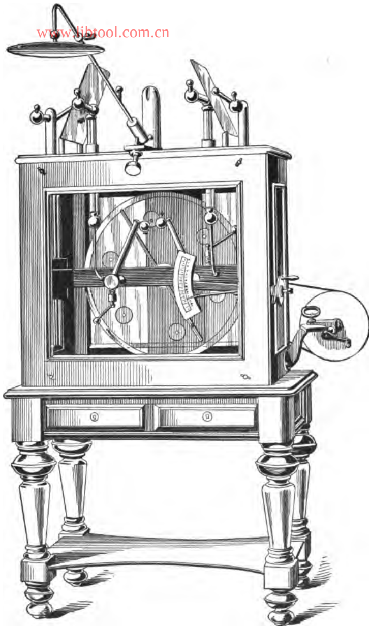
FIG. 89.—HOLTZ-TOEPFLER MACHINE.—( Hirschmann, Berlin. )
