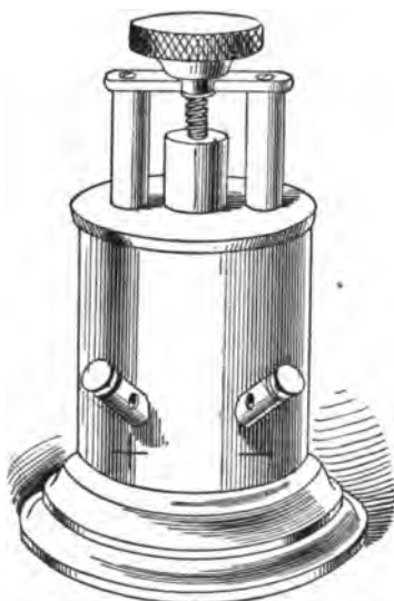
FIG. III.—FLUID RHEOSTAT.
