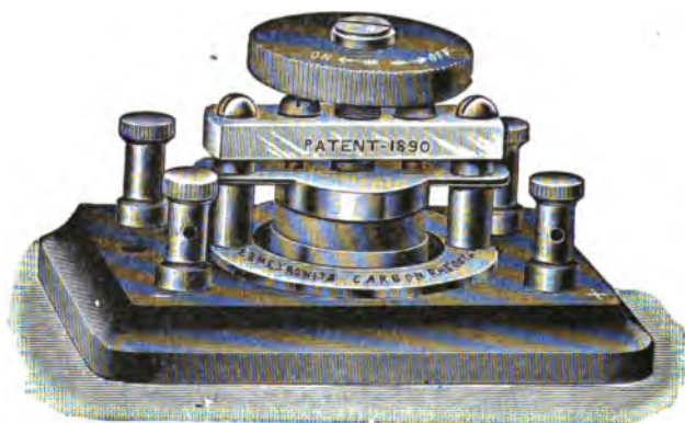
FIG. 109.—VETTER RHEOSTAT.
