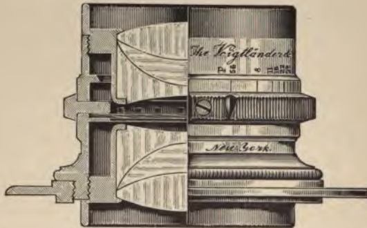
FIG. 13. "Collinear" Lens. Voigtländer & Son Optical Co.
