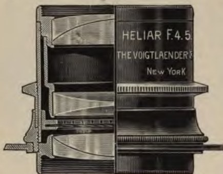
FIG. 42. "Heliar" Lens. Voigtländer & Son Optical Co.
