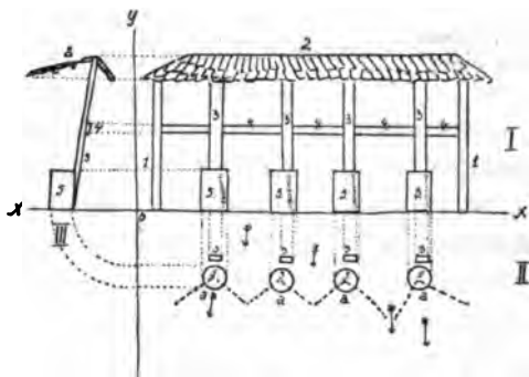
136. Strunka . I. Widok z przodu. 1. paluch; 2. powirchnyk; 3. deski; 4. pobedryna; 5. siedaki. Strzały wskazują, którądy owce przechodzą, a... położenie kolan juhasów. II. Przekrój poziomy strunki; oznaczenia jak w I. nadto a owce przy podoju. III. Przekrój boczny.
