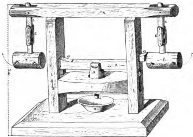
106. Olejnica . 1. kołoda; 2. cówka; 3. słupy; 4. prawyło; 5. skrakli; 6. skraknyki; 7. tarany; 8. strilá z zájacem; 9. i 10. klyný; 11. misa.
