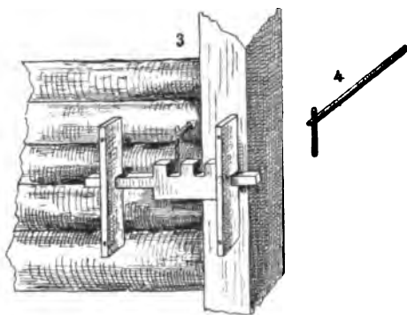
39. Zamek odnorucnyj . 3. pozioma zasuw, wysunięta z po za drzwi, spoczywa w dwu pionowych odźwiernikach; przez dziurę w zrębie włożony klucz, którego język wpadł w karb zasuwu. 4. Klucz osobno.
