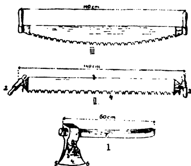
119. I. Siekiera . 1. obúch; 2. pazuchý; 3. szyja; 4. pleczé z wístríem, które ma nosók 5, i boridku *6; 7. toporzysko. II. Pyła práwa . 1. rucz-nýcia; 2. ruczký; 3. chřebet; 4. zubáte wístríe. III. Pyła kalucháta .
