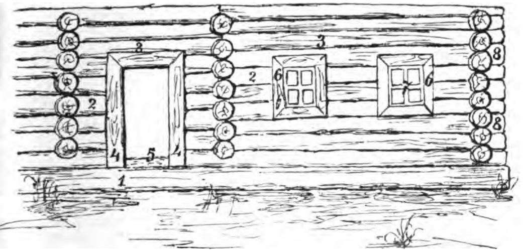
32. Zrąb, ostręb . 1. podwalina; 2. sumik, soméc ; 3. leżuch, prawyło ; 4. odrzwi; 5. próg; 6. warcaby; 7. ramki; 8. węgły.
