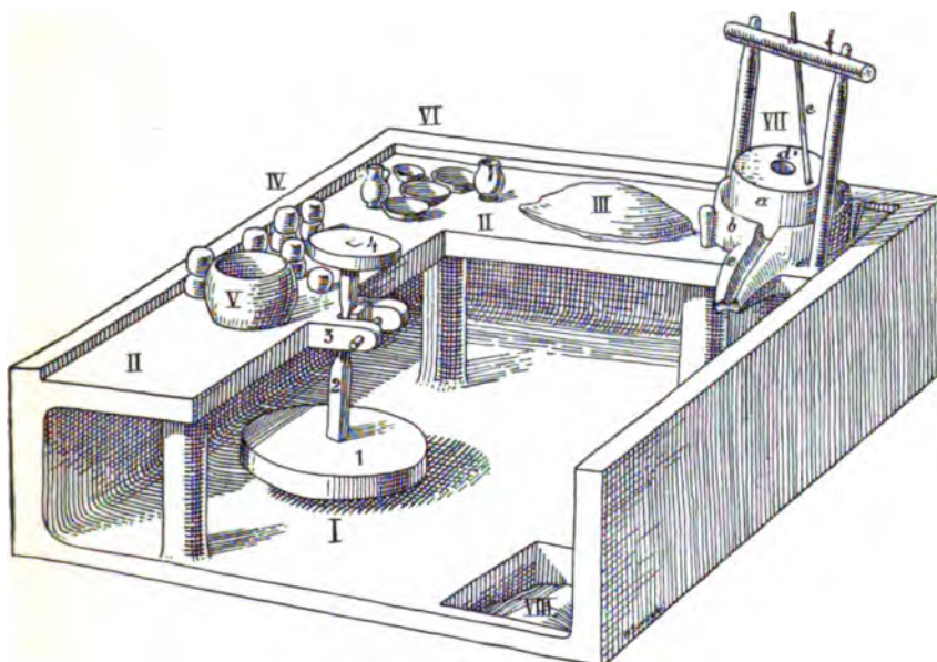
181. Garncarski warstat. I. Kruh . 1, spidnyk ; 2, vereteno ; 3, zabky . 4, verchniak . — II. Ławka. — III. Glina przygotowana do miszenia. — IV. Grudki już wymieszanej gliny. — V. Miska z wodą. — VI. Wyro-bione naczynie. — VII. Żarna. a. kamień; b. obręcz; c. pręt; d. gardło; e. żłódek; f. krosna. — VIII. Jama z gliną.
