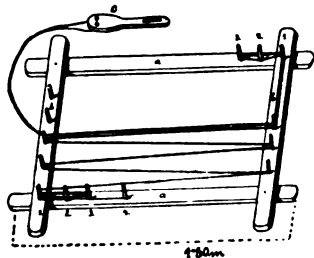
99. Snuwánka . a) pobédryny ; b) kołúdrabky ; 1. 2. 3. 4. czopy ; c) snuwánnyk .
