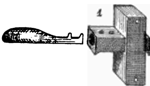
38. Zamek ławcziestyj . 1. Klucz wyciągnięty z poziomej zasuw umieszczonej w pionowym odźwierniku. 2. Przekrój przez zamknięty zamek; zasuw zasunięta, w jej otwory powpadały ławki , do których klucz zębami przytyka.
