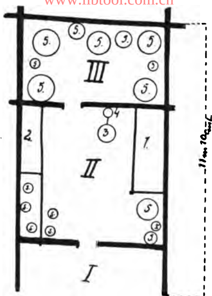
131. Plan staj 130. I. Poddásze. II. Watarnyk. III. Komóra. 1. 2. ławki; 3. watra; 4. werkluh; 5. bodnie i t. p.
