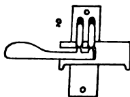
38. Zamek ławcziestyj . 1. Klucz wyciągnięty z poziomej zasuw umieszczonej w pionowym odźwierniku. 2. Przekrój przez zamknięty zamek; zasuw zasunięta, w jej otwory powpadały ławki , do których klucz zębami przytyka.
