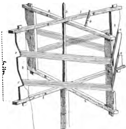
98. Samotóka . 1. 2. jérma ; a) perechrésnyci ; b) kaczki ; c) zázuby . 3. swóreń ; 4. rozhin .
