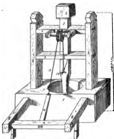
105. Pochodźnica stupa . 1. kołoda; 2. stow; 3. nóżne- 4. wężne prawyło; 5. makohin; 6. głowa; 7. żieb- kły; 8. wał u żiebkach; 9. podnóża; 10. łabkły; 11. wał; 12. stúpateń; 13. sznur, przechodzący rynienkę w obwodzie kółka a przywiązany do klúka 14.
