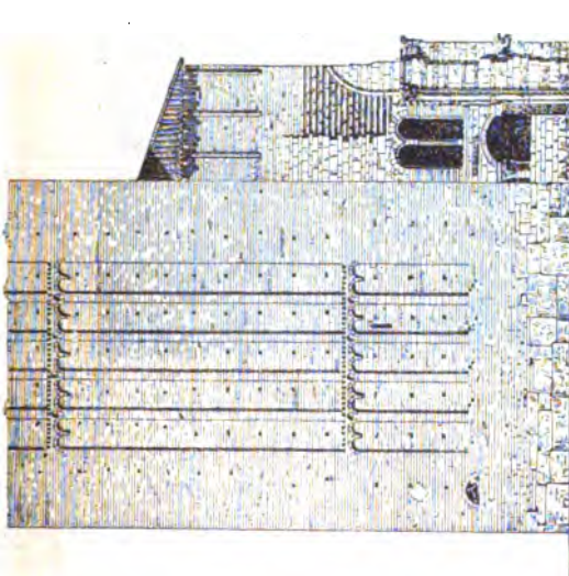
COLLOCAMENTO DEI FRANGENTI DELLA DISTRUTTA BASILICA DI SANTO STEFANO DI PAVIA
