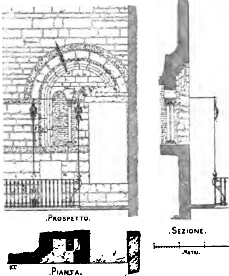
·PALAZZO DEL BROLETTO. BRESCIA· ·COME FU TROVATA VNA DELLE FINESTRE TRIFORE SULL· LATO DEL CORTILE RIVOLTO A TRAMONTANA DOPO GLI· ASSAGGI FATTI NEL DICEMBRE DEL 1892.
