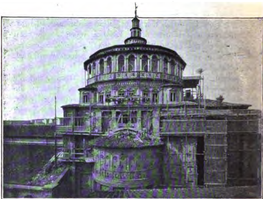
CUPOLA DELLA CHIESA DI S. MARIA DELLE GRAZIE (durante il restauro).
