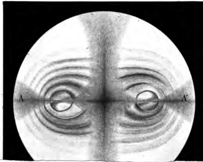
Fig.1. Dispersion croisée. Lame taillée perpendiculairement à la bissectrice argüe, placée de manière que AA' soit à 45^\circ de la vibration du polariseur.
