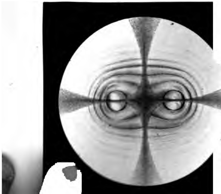
Dispersion horizontale à l'axe optique parallèle à la bissectrice
