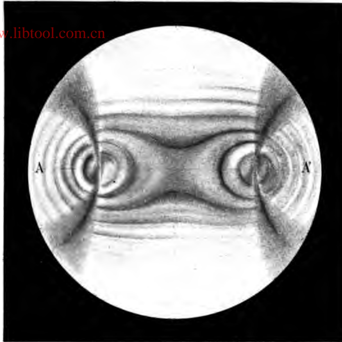
Fig.1. Dispersion croisée. Lame taillée perpendiculairement à la bissectrice argüe, placée de manière que AA' soit à 45^\circ de la vibration du polariseur.
