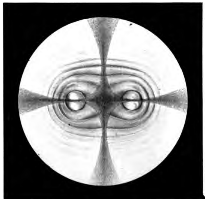
Fig. 2. Dispersion horizontale. Même lame que dans le triangle ci-dessus, placée
