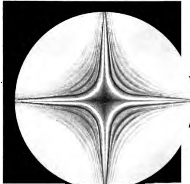
Fig.1. Cristal biaxe , taillé perpendiculairement à un axe optique vu entre deux nicols croisés, la ligne des pôles AA' étant parallèle à l'une des vibrations du polariseur ou de l'analyseur.
