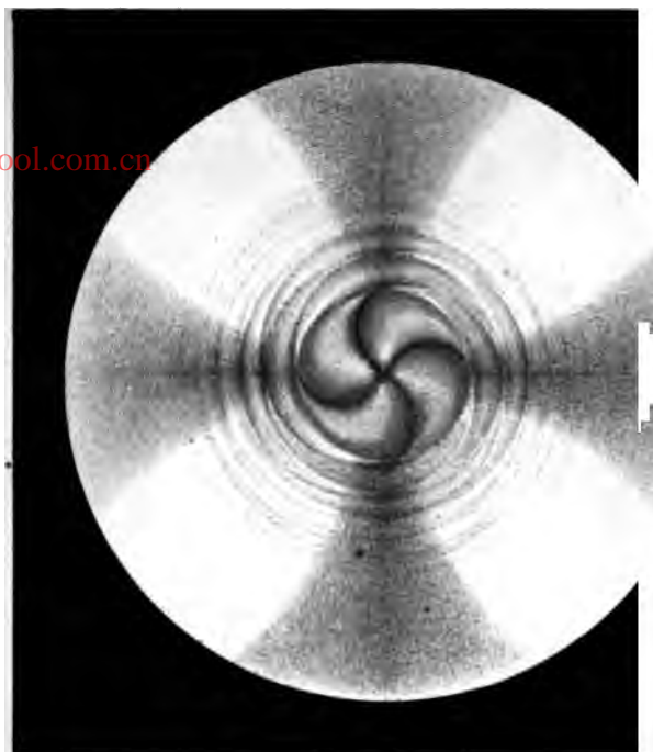
Fig. 1. Deux lames de quartz superposées, d'égale épaisseur et de rotation inverse, la lame dextrogyre étant au-dessous.
