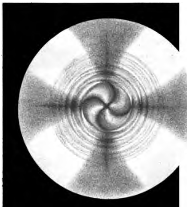
Fig. 2. Deux lames de quartz superposées, d'égale épaisseur et de rotation inverse.
