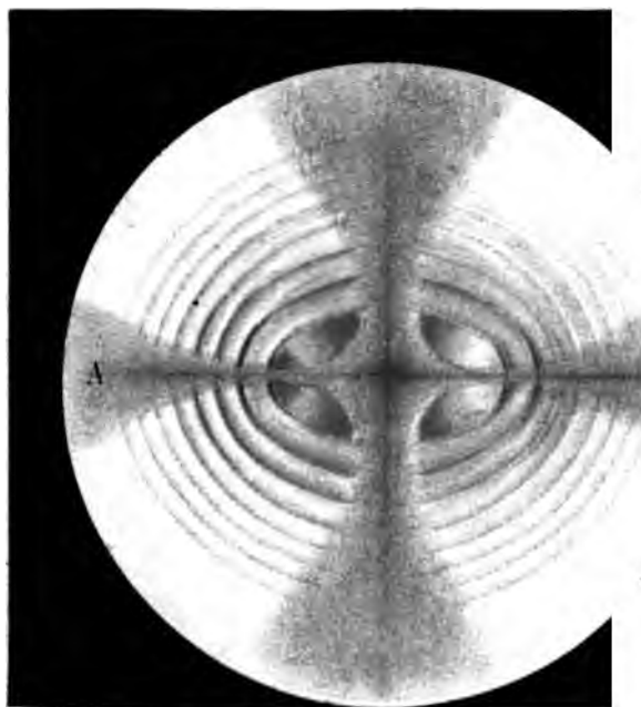
Fig.1. Dispersion inclinée. Lame taillée perpendiculairement à la bissectrice, est placée de manière que AA' soit à 45° de la vibration du pol.
