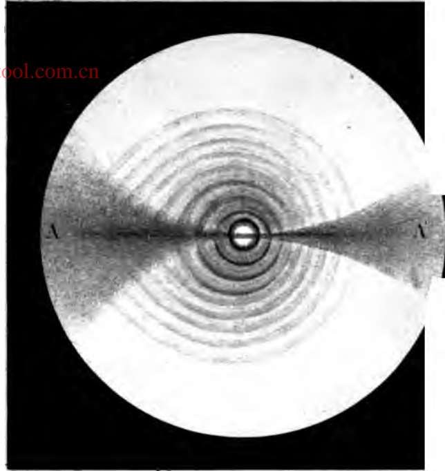
Fig.1. Cristal biaxe , taillé perpendiculairement à un axe optique vu entre deux nicols croisés, la ligne des pôles AA' étant parallèle à l'une des vibrations du polariseur ou de l'analyseur.
