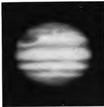
FIG. 12.—JUPITER
