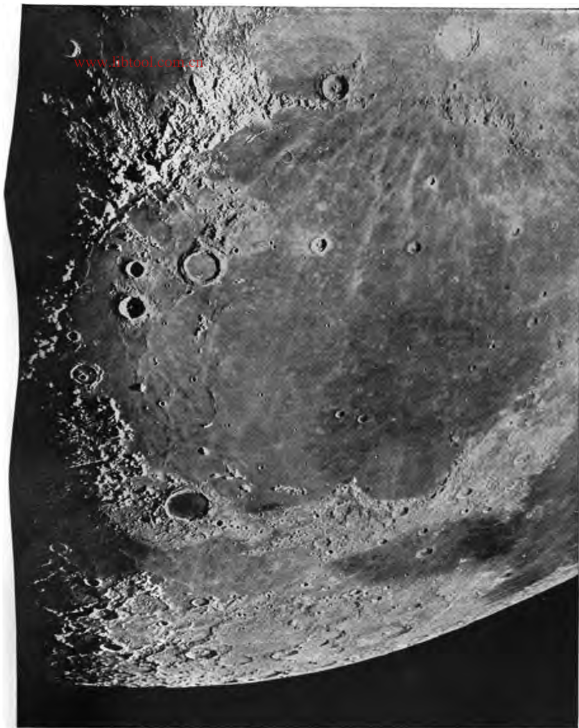
FIG. 14.—THE MOON
