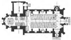
Perspektivische Ansicht von Nordosten und Grundriss.
