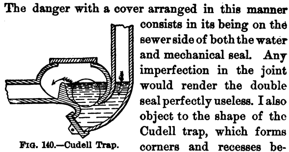
FIG. 140.—Cudell Trap.
