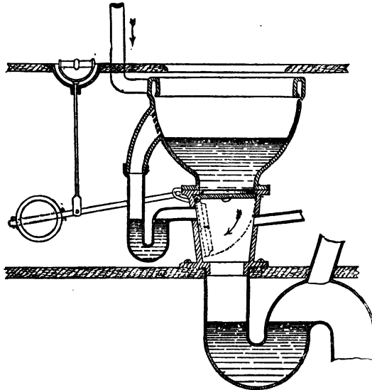
FIG. 12.—Valve Closet.
