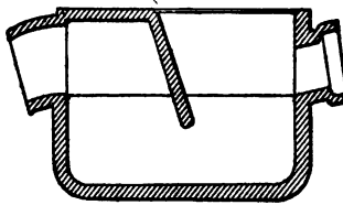
FIG. 56.—Bavin Trap.
