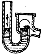
FIG. 142.—Buchan's Trap.
