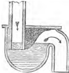
FIG. 5.—D-Trap.
